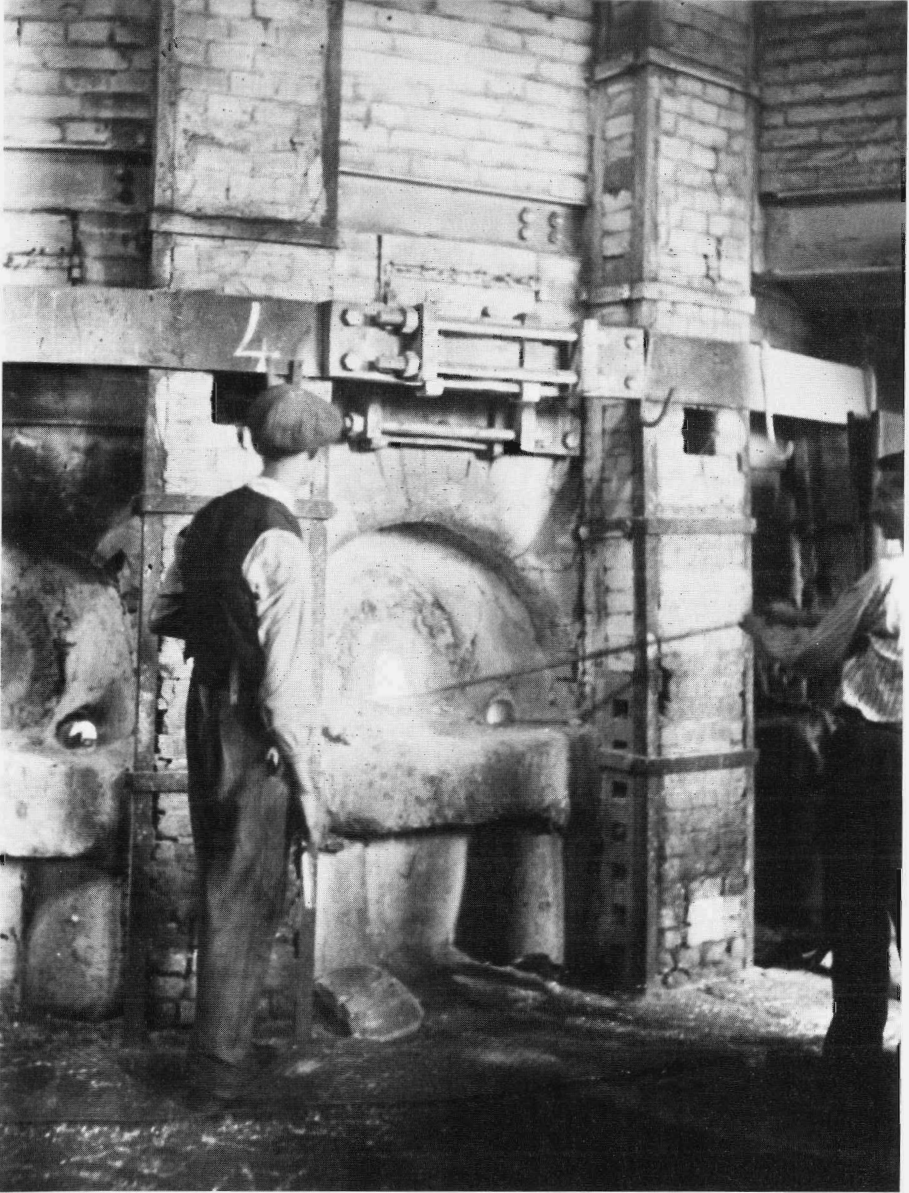
De voorvormer (carreur) neemt een hoeveelheid glas uit de werkopening van een smeltoven en draait dat op het einde van een ijzeren holle buis rond. Hij blaast een beetje lucht in de buis en geeft die met glas vervolgens door aan een van leerjongens (gamins).
