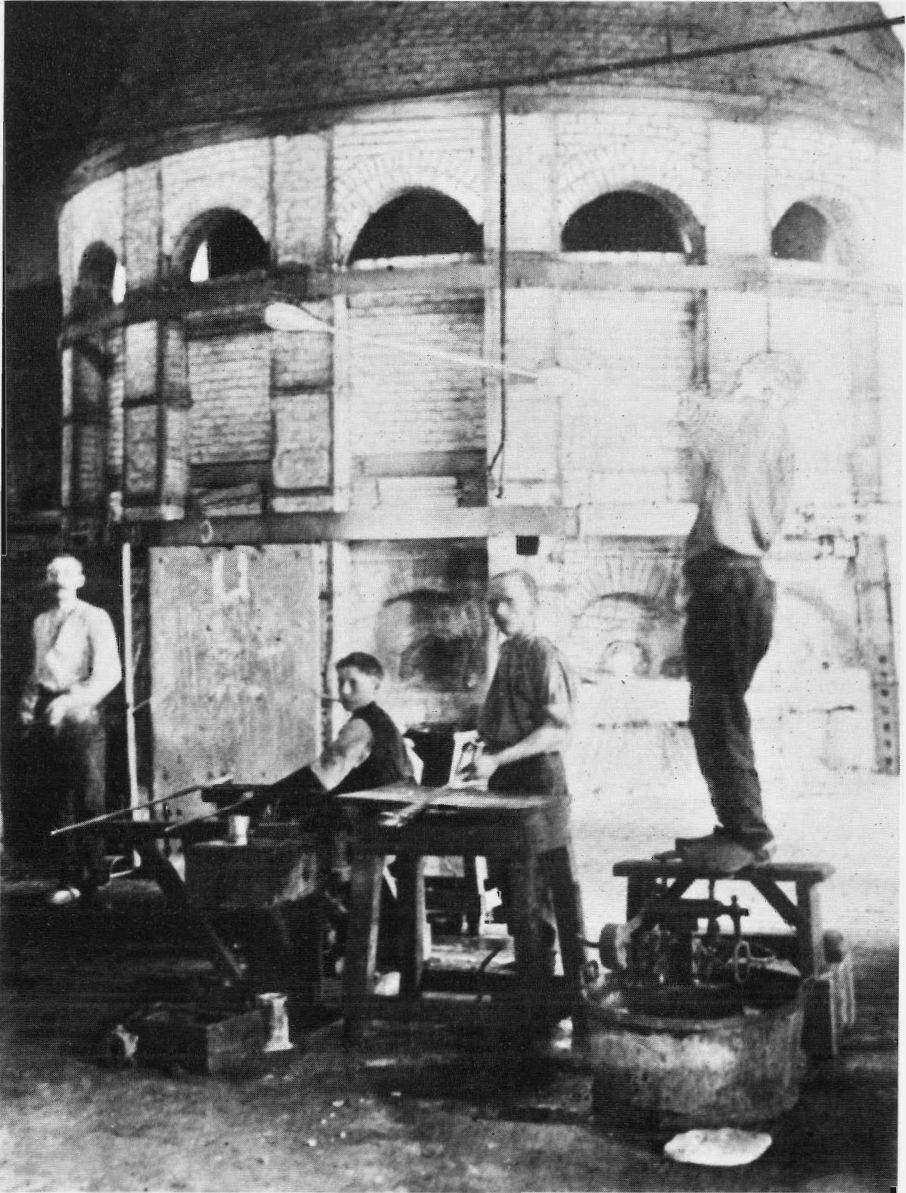
De werkmán (ouvrier) achter de tafel rolt een ijzeren buis met glasklomp over de tafel, terwijl de glasblazer (souffleur) staande op een trapje een flesvormig voorwerp blaast.
