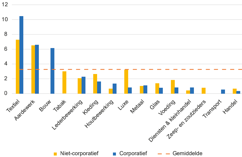
Grafiek 1 Arbeidsverhoudingen (O/M) per sector naargelang corporatieve organisatie, nijverheidsenquête (1738) – selectie van 9 steden
